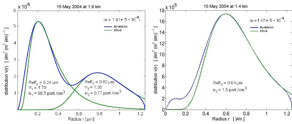
Fig. 2. Microphysical parameter retrieval on 15 May 2004.
